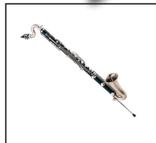
clarinete bajo
