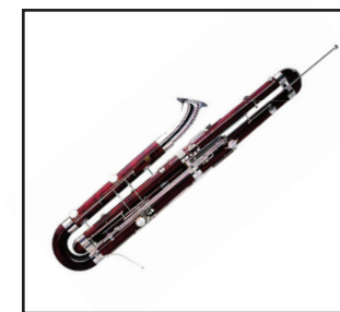
contrafagot
