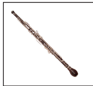
corno inglés
